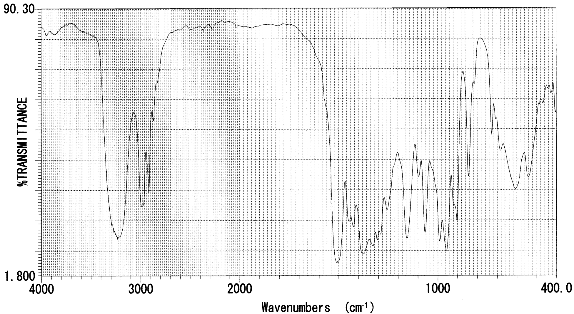
品名：1-メチルエチレンビスジチオカルバミン酸ジメチル標準品 測定条件：液膜法
