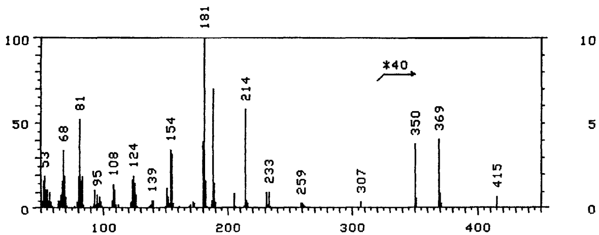
MSスペクトル
