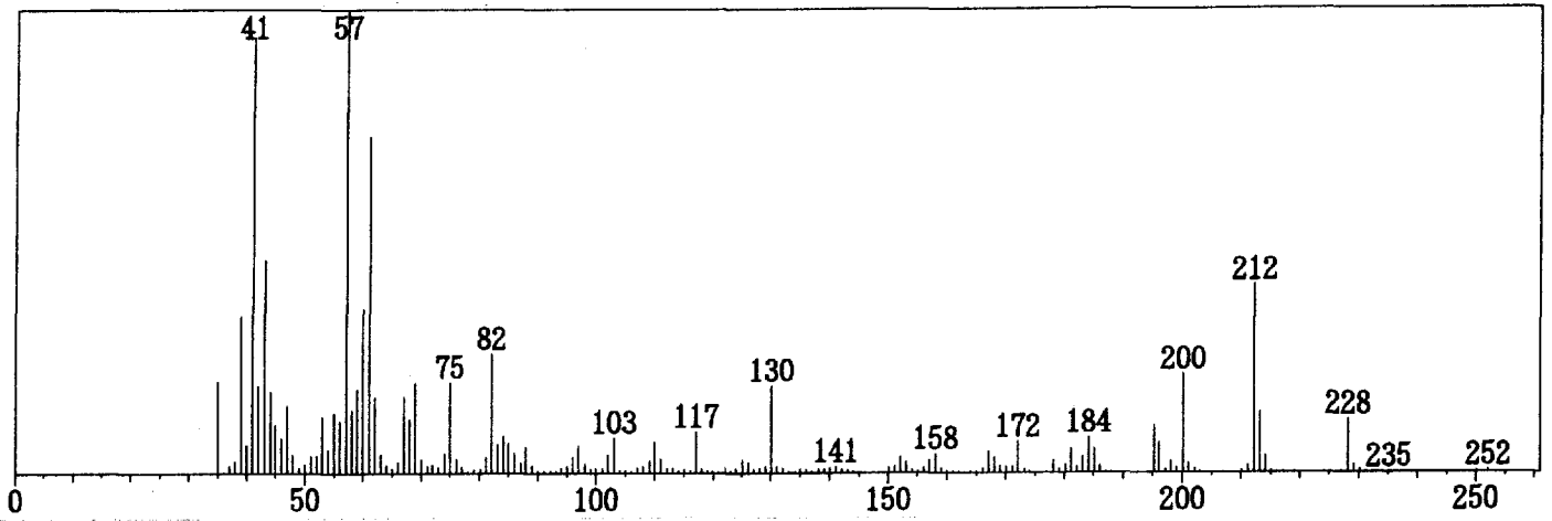
MS スペクトル
