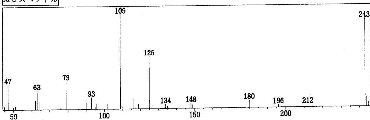
MS スペクトル
