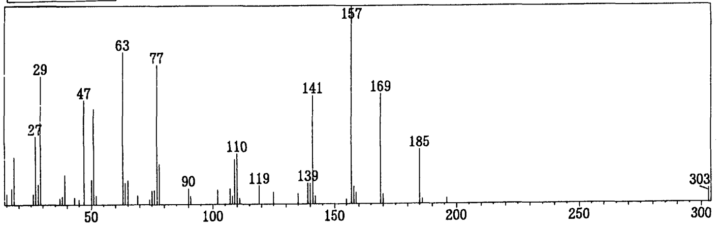
MS スペクトル
