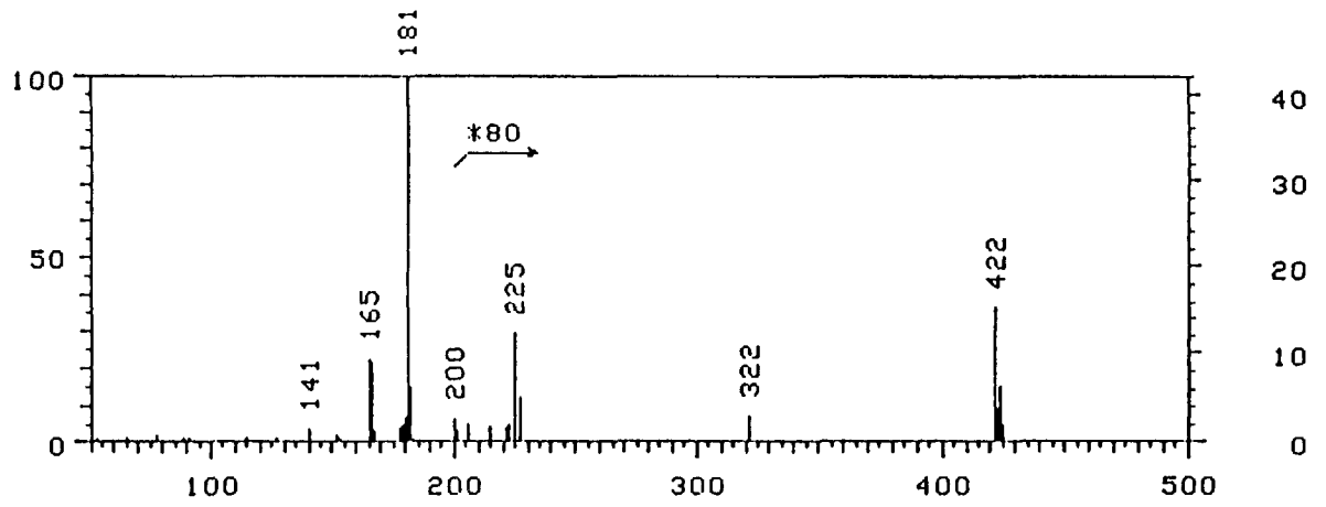
MSスペクトル
