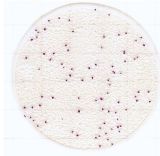
Saccharomyces cerevisiae
