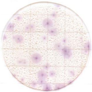
Aspergillus flavus
