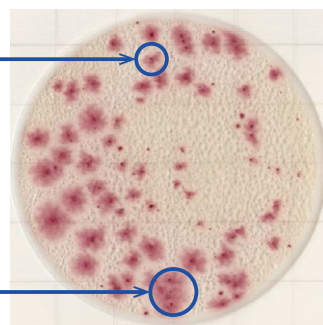
Pseudomonas aeruginosa
